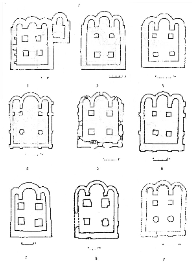
Рис. 7. Сводная таблица планов некоторых древнерусских храмов (по Вл. В. Седову):
