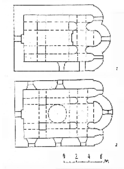
Рис. 9. Собор Св. Иоанна Богослова Черемнецкого монастыря Планы подцерковья (1) и храма (2) (по Вл. В. Седову, элементы реконструкции – автора)
