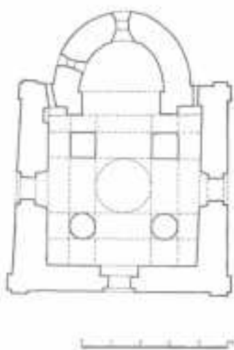
Рис. 4. Церковь Рождества Богородицы в Порхове Реконструкция плана (по Вл. В. Седову)
